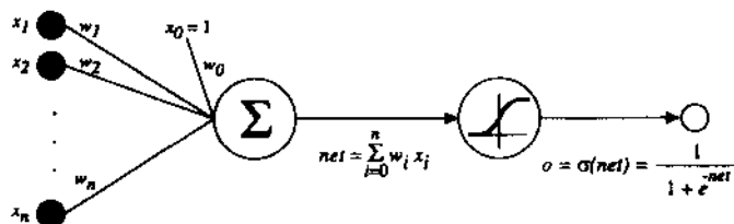
图 4-6 sigmoid 阈值单元
