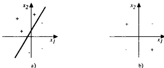
a)一组训练样例和一个能正确分类这些样例的感知器决策面, b)一组非线性可分的训练样例(也就是不能用任一直线正确分类的样例)。 x_1 和 x_2 是感知器的输入,“+”表示正例,“-”表示反例
