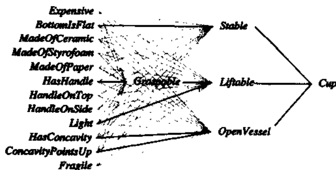
这个网络在 KBANN 算法的第一阶段创建出来,它产生的输出分类等于给定的领域理论中的子句做的分类。粗线表示权值为 W 的连接,对应领域理论中的子句先行词。细线表示权值近似为 0 的连接
