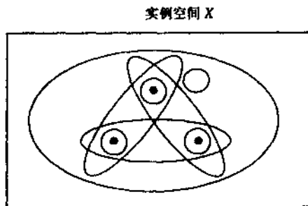
图 7-3 被 8 个假设拆散的包含 3 实例的集合
