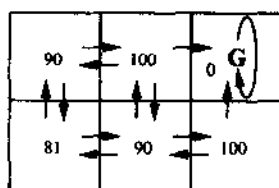
V^*(s) 值
