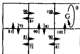
Q(s, a) 值
