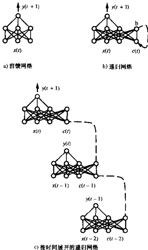
图 4-11 递归网络
