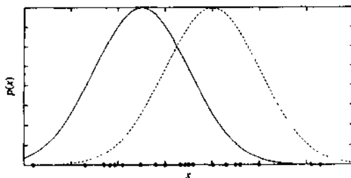
实例为沿着 x 轴显示的点集。如果正态分布的均值未知,EM 算法可用于搜索其极大似然估计
