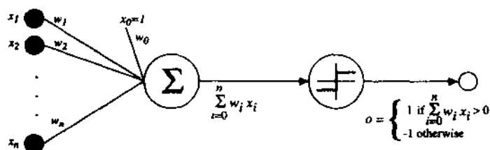
图 4-2 感知器
