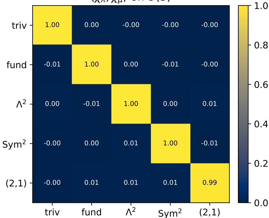
\langle \chi_\lambda, \chi_\mu \rangle on U(3)
