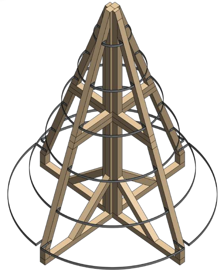
PŘIPRAVENÁ KONSTRUKCE (na pásovinu se poté přidělají došky těsně vedle sebe)
