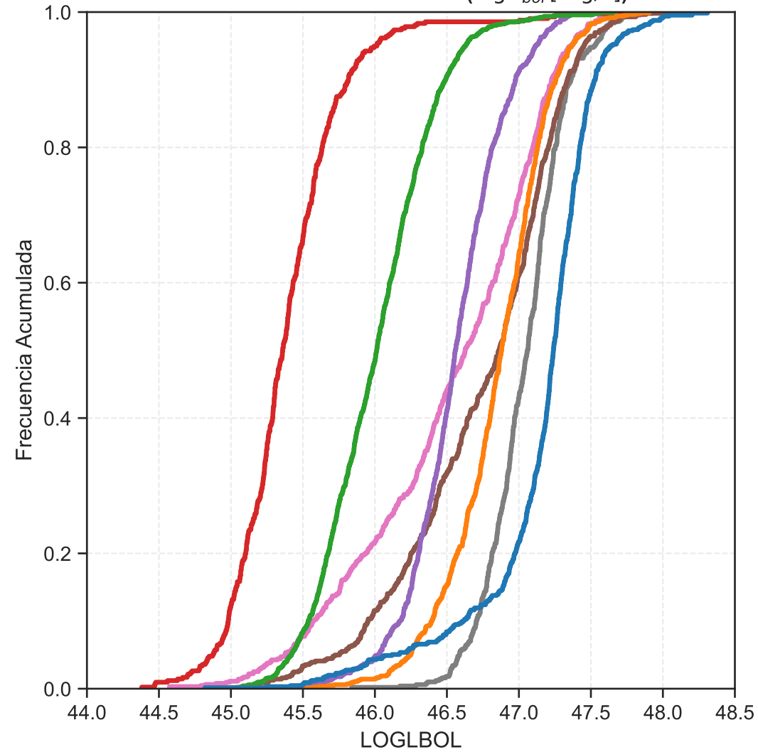
Luminosidad Bolométrica ( \log L_{bol} [erg/s])
