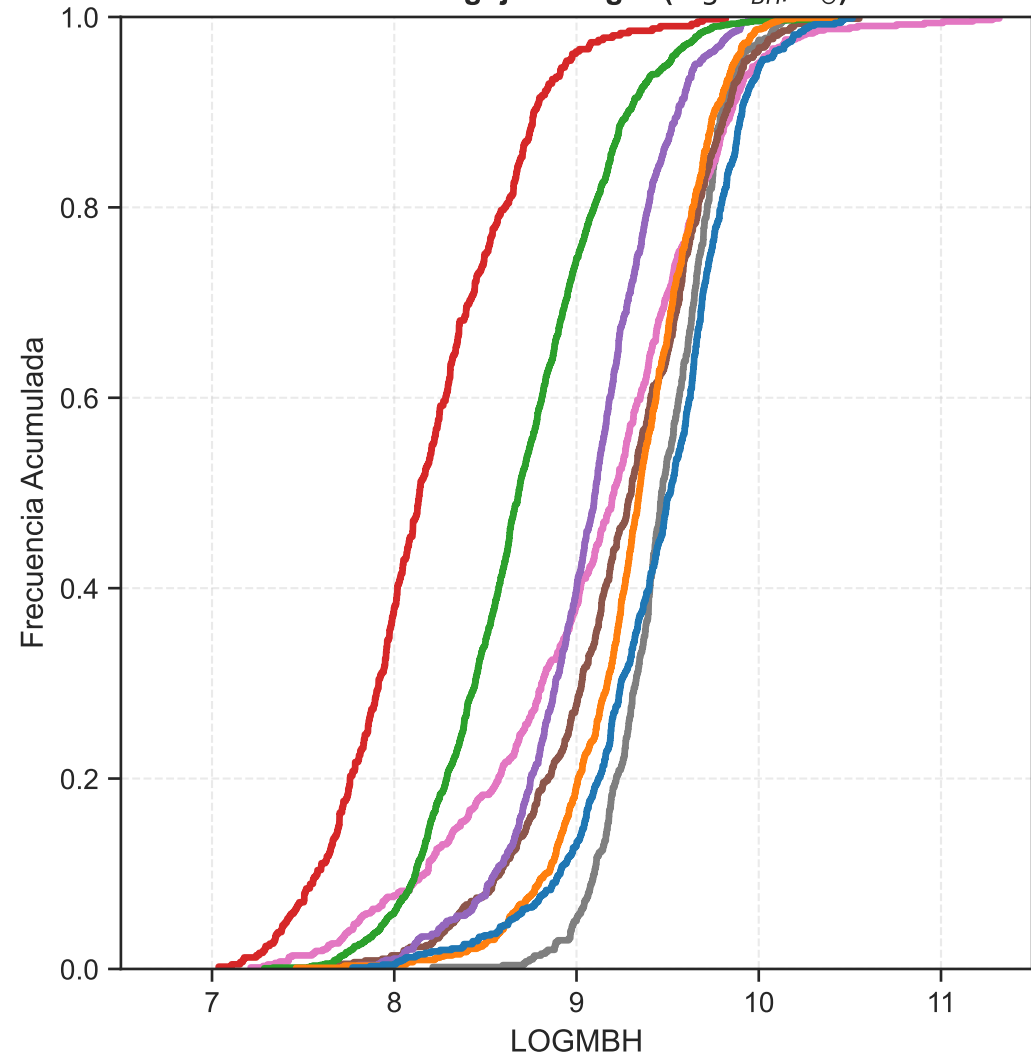
Masa del Agujero Negro ( \log M_{BH}/M_{\odot} )
