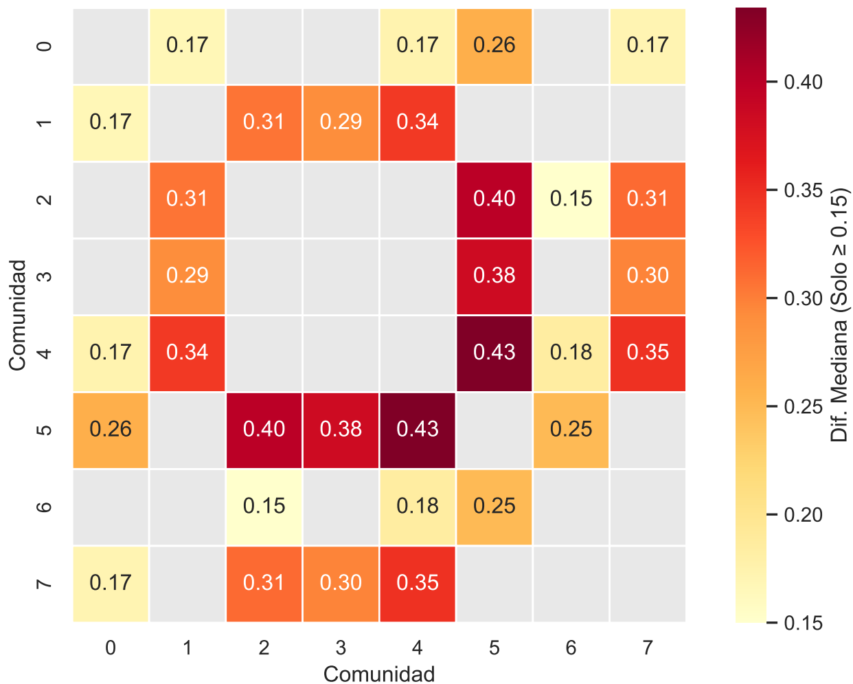
Matriz de Supervivencia: h_k (Filtro: p < 0.05 , Cliff \geq 0.33 , \Delta \geq 0.15 )
