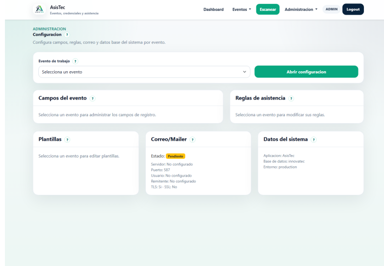
Modulo Configuracion.
