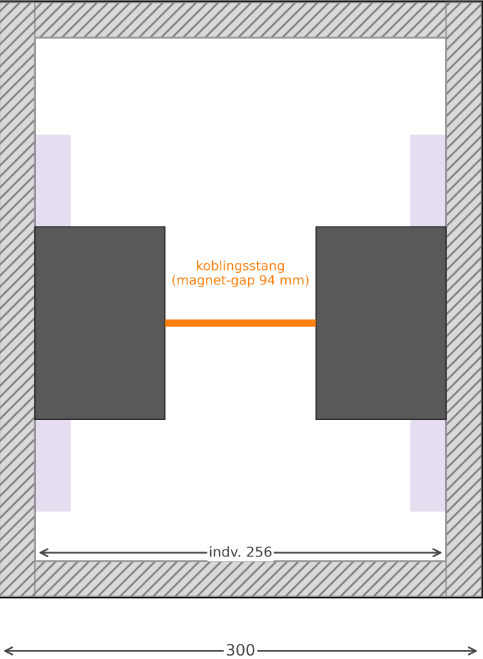
Snit B-B - gennem basserne (push-push)
