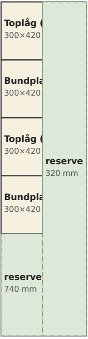
Plade 5 toplåg + bund
