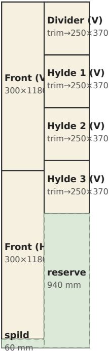
Plade 3 front + div V + hylder V
