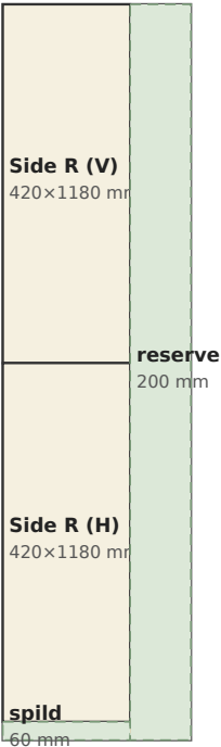
Plade 2 sider H
