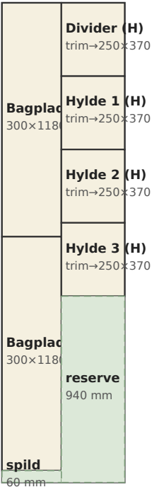
Plade 4 bagplade + div H + hylder H
