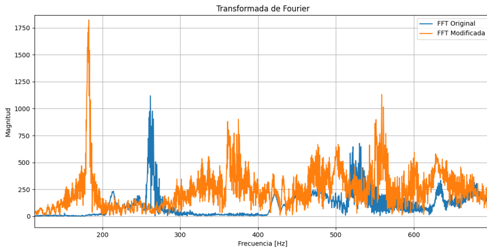
Figura 32: Transformada de Fourier de la señal original y modificada.
