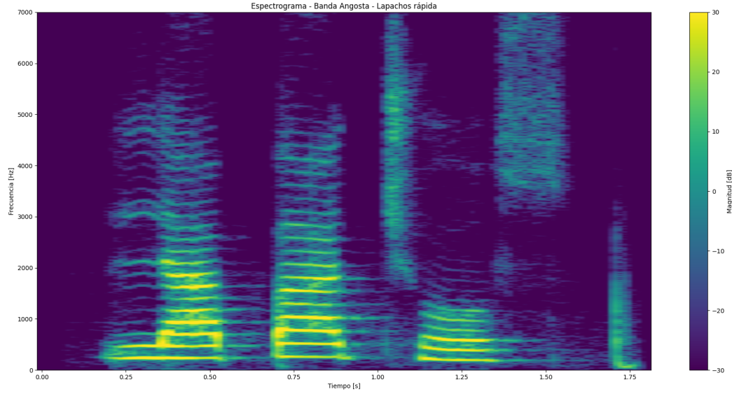
Figura 43: Espectrograma de banda angosta de Lapachos rápida.
