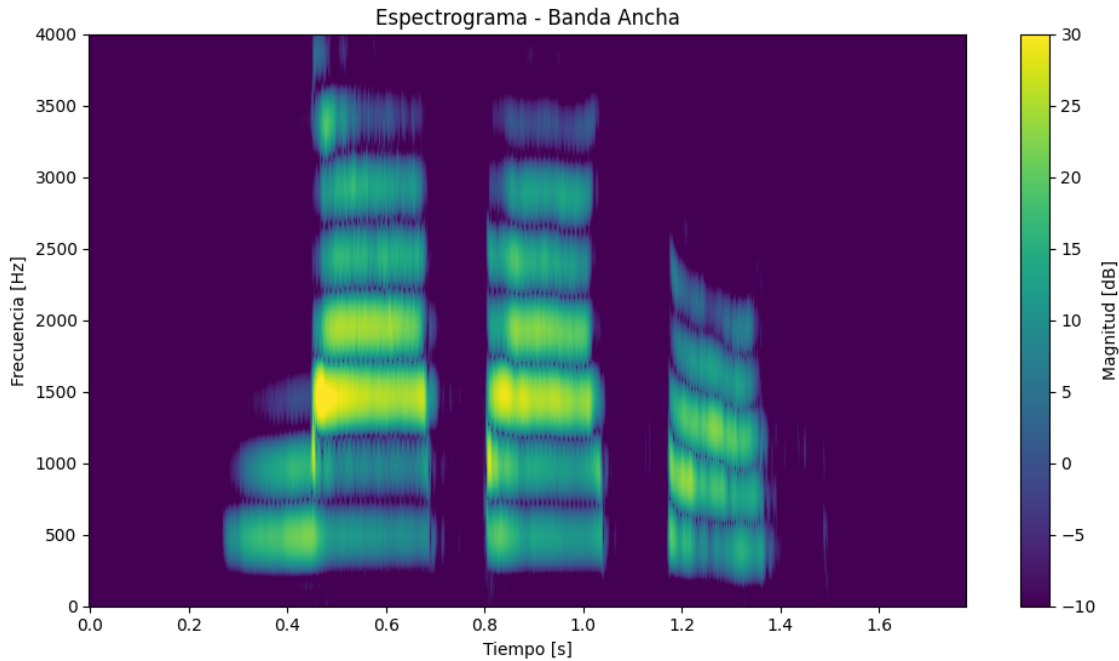
Figura 36: Espectrograma de banda ancha de Lapachos lento decimado.
