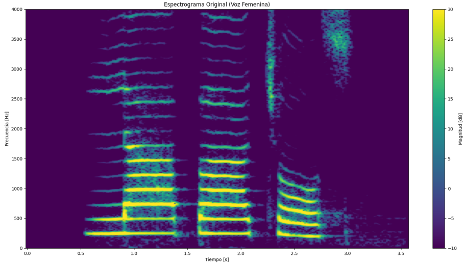
Figura 34: Espectrograma de banda angosta de la señal original.
