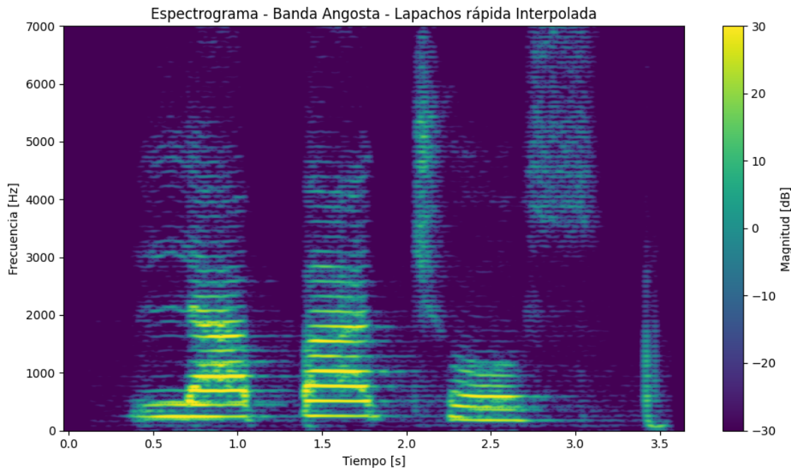
Figura 42: Espectrograma de banda angosta de Lapachos rápida procesada.
