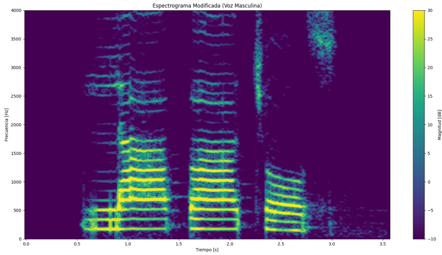
Figura 35: Espectrograma de banda angosta de la señal modificada.
