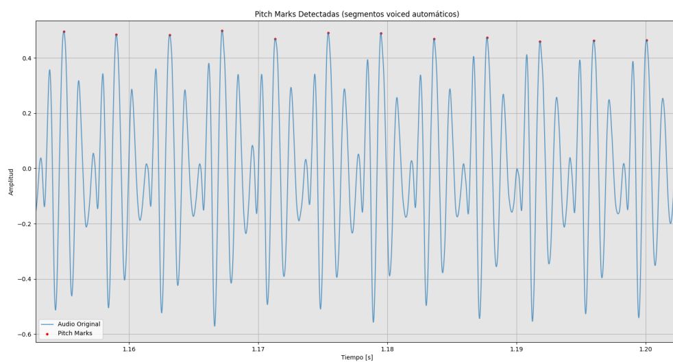
Figura 32: Pitch marks sobre tramo cuasiperiódico de Lapachos lenta.
