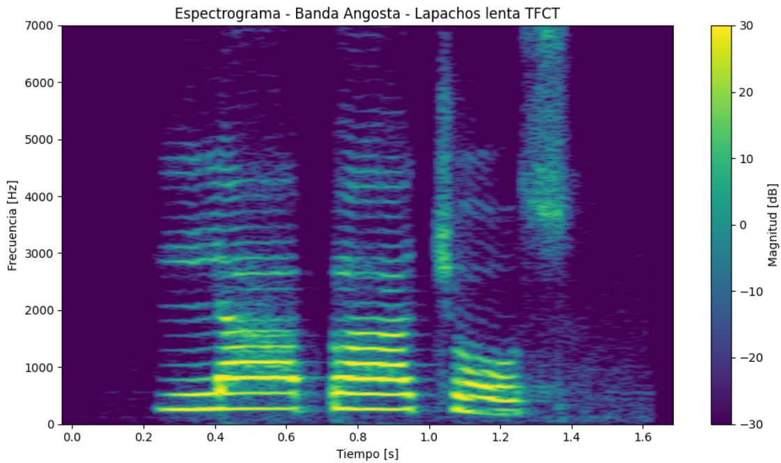
Figura 40: Espectrograma de banda angosta de Lapachos lenta procesada.
