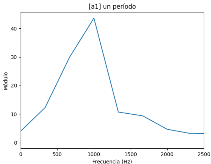
Figura 14: FFT Letra [A1] - Un período - señal lenta.
