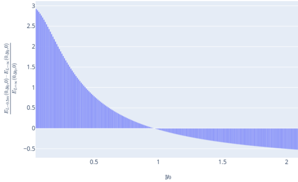
Figure 6: Diferencias percentuales entre el uso de L = 0.5m y L = \infty (i.e., \frac{E_{L=0.5m}(0, y_0, 0) - E_{L=\infty}(0, y_0, 0)}{E_{L=\infty}(0, y_0, 0)} ). Haga click en la imagen para ver su version interactiva. El código usado para construir esta figura se encuentra aquí .
