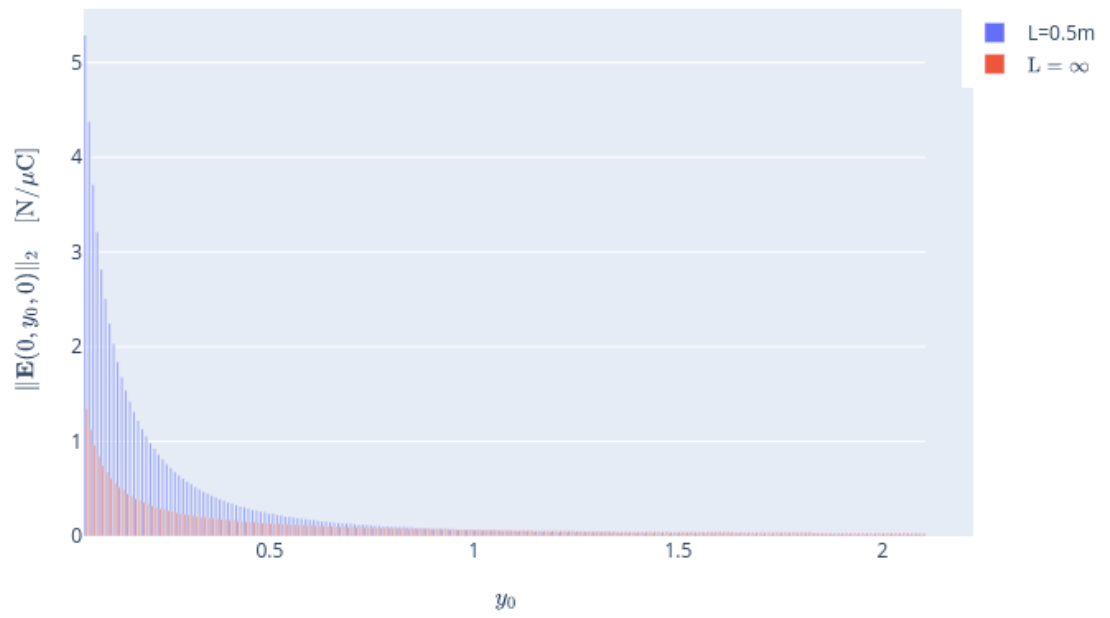
Figure 5: \|E(0, y_0, 0)\|_2 en function de y_0 , usando \lambda = 15\mu C/m y L = 0.5m (barras azules) o L = \infty (barras rojas). Haga click en la imagen para ver su version interactiva. El código usado para construir esta figura se encuentra aquí .
