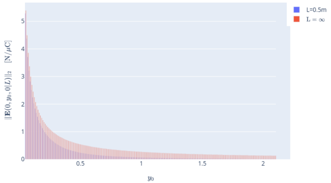
Figure 5: \|E(0, y_0, 0)\|_2 en función de y_0 , usando \lambda = 15\mu C/m y L = 0.5m (barras azules) o L = \infty (barras rojas). Haga clic en la imagen para ver su versión interactiva. El código usado para construir esta figura se encuentra aquí .
