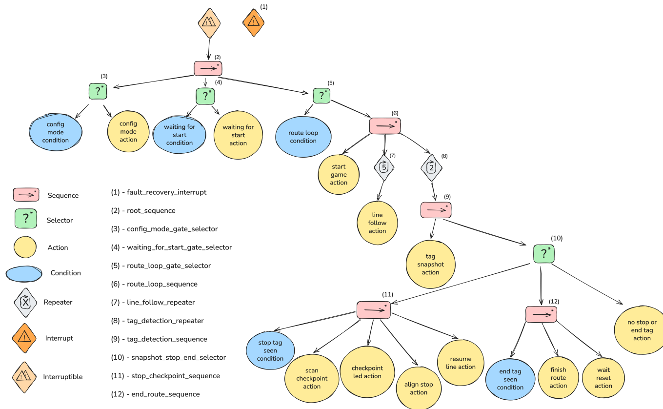
Figura 4.2: Árbol de comportamiento implementado en Robotito.
