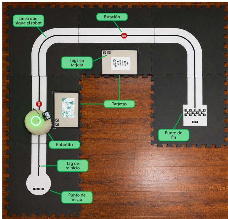
Figura 1.1: Montaje completo de la actividad. En la imagen se pueden observar el tablero modular, la línea que sigue Robotito durante el recorrido, el propio Robotito, los tags de referencia utilizados para detener o guiar la ejecución, las estaciones donde se ubican las tarjetas, y las tarjetas con dibujos colocadas por los estudiantes. También se observan el punto de inicio y el punto de fin del recorrido.
