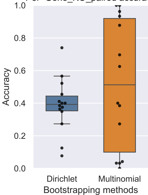
Per-Gene_KO_pair accuracy
