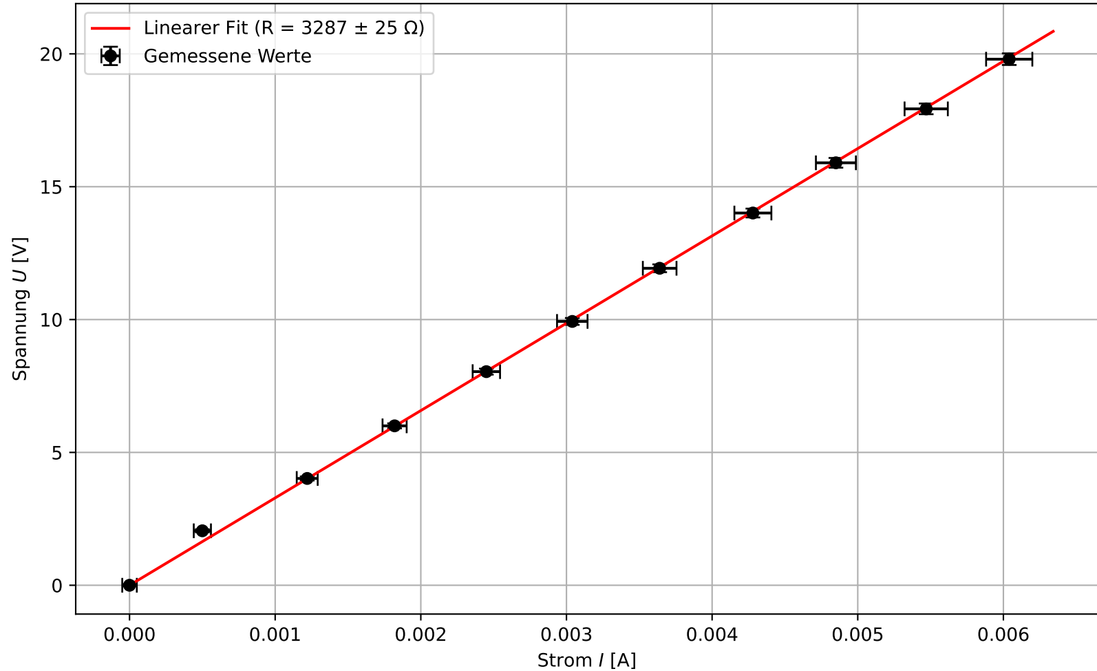
U-I Diagramm zur Bestimmung des Widerstands
