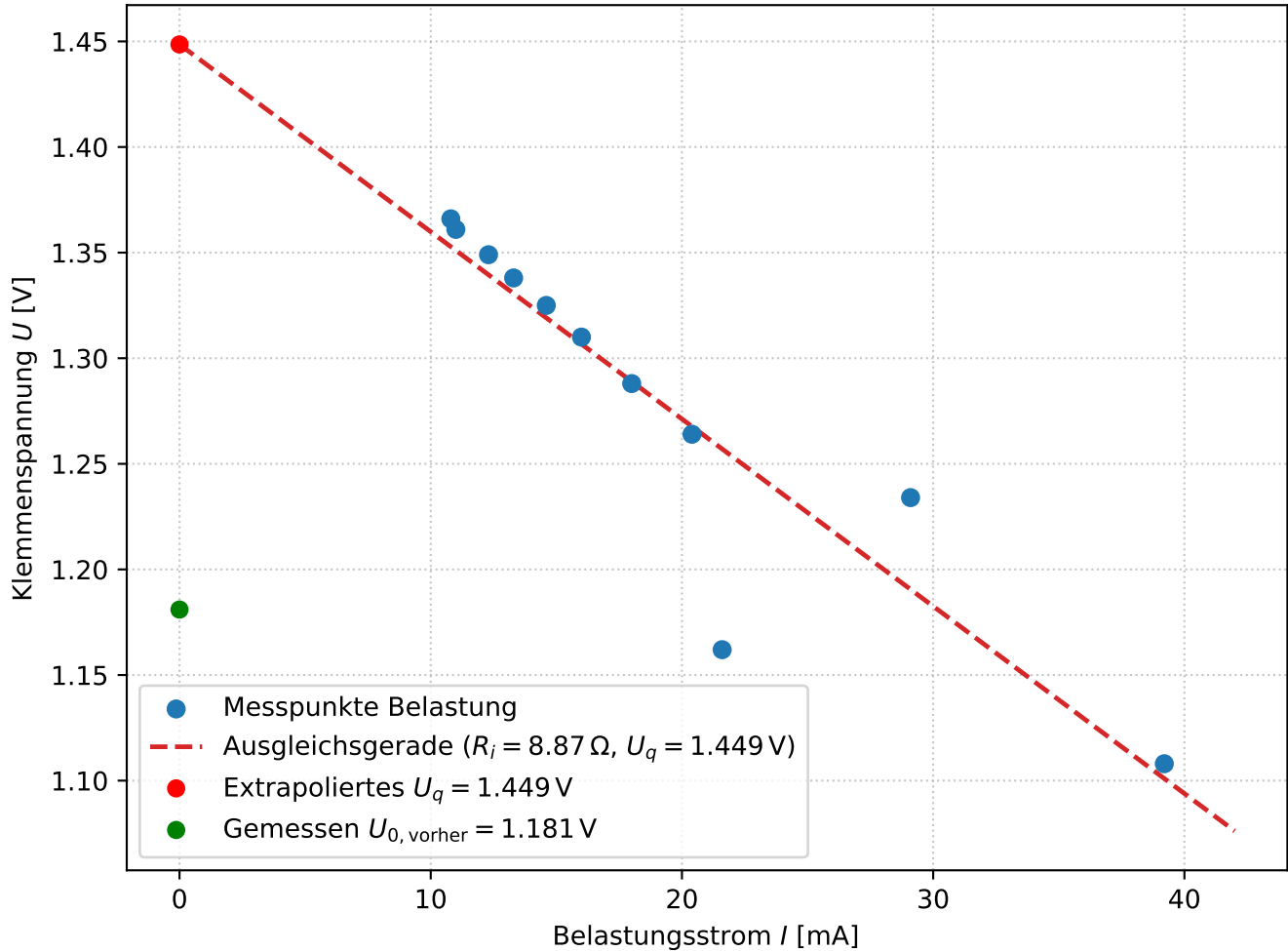
Belastungskennlinie der galvanischen Zelle
