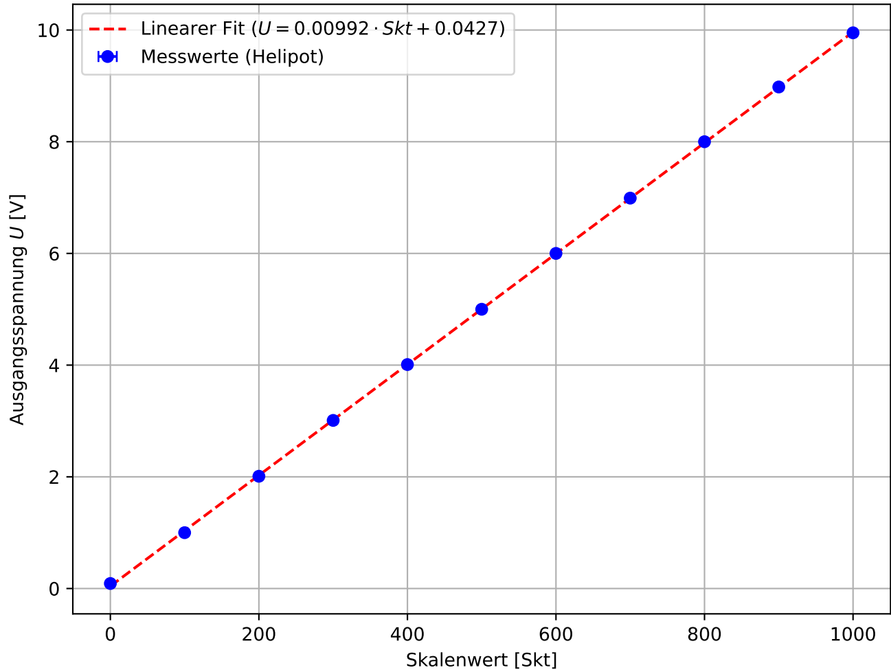
Ausgangsspannung des Helipot gegen Skalenwerte
