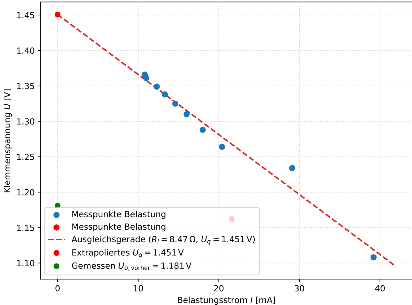
Belastungskennlinie der galvanischen Zelle
