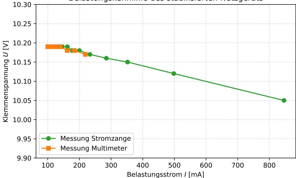
Belastungskennlinie des stabilisierten Netzgeräts
