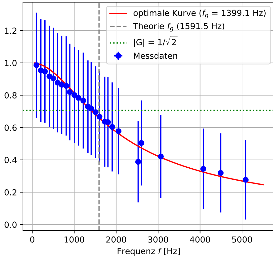
Tiefpass
