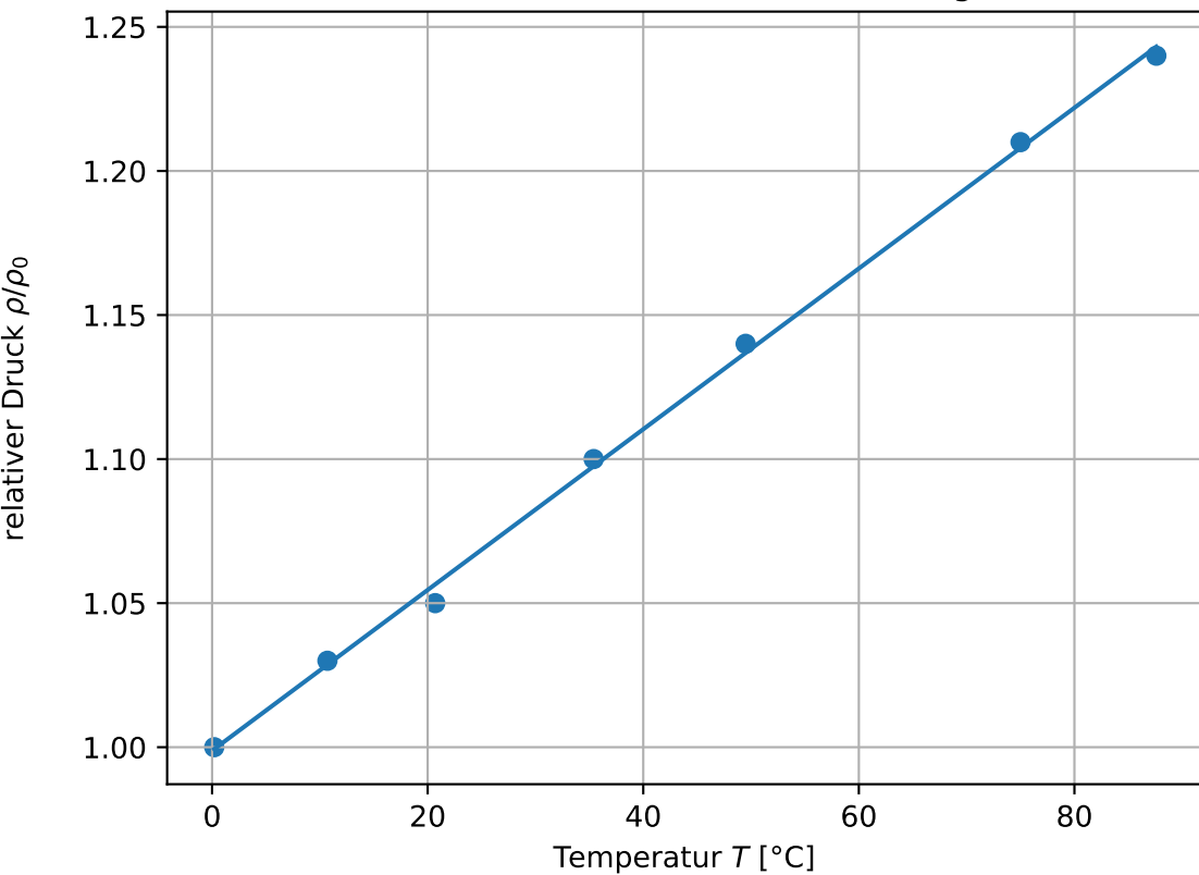
TV2: Isochore Zustandsänderung
