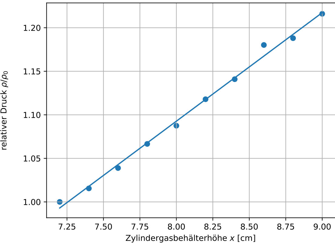
TV1: Isotherme Volumenexpansion ( T_0 = 88,3 \pm 0,05^\circ\text{C} )
