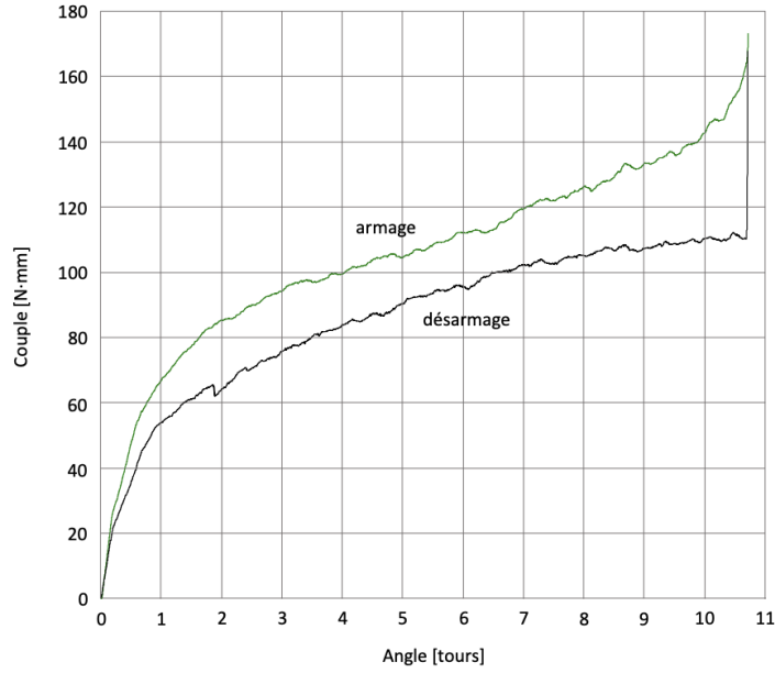
Figure 20: Couple d'armage et de désarmage du barillet en [\text{N}\cdot\text{mm}] en fonction du nombre de [tours]
