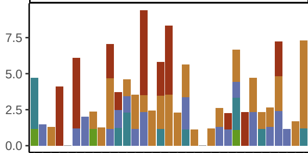
EBV.nasal
