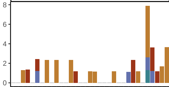
CMV.nasal
