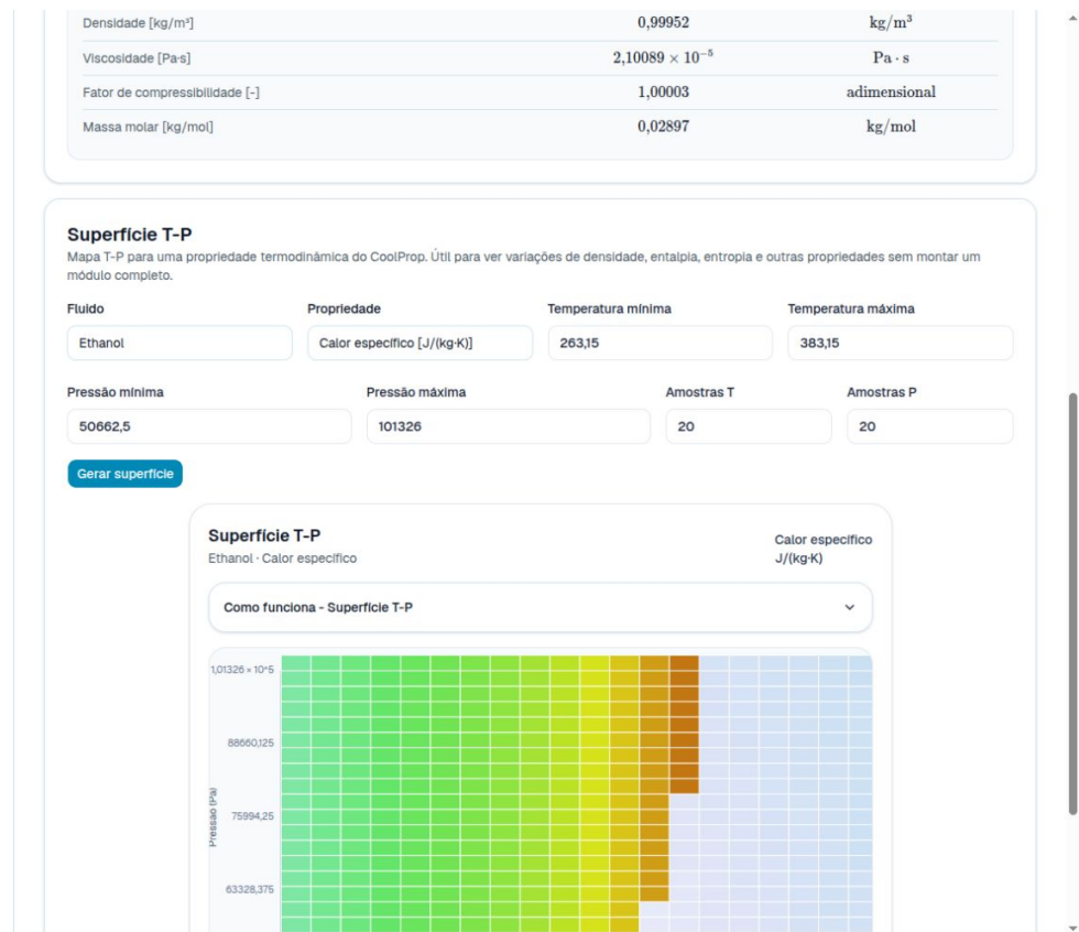
Figura 76 – Aba Fluido Puro com propriedades e superfície T-P
