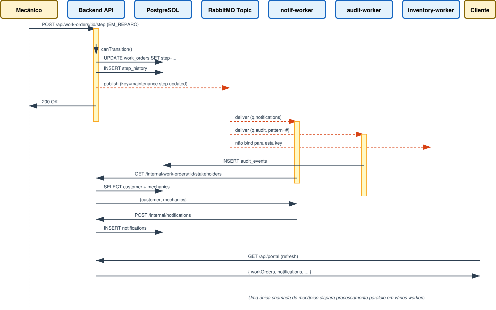
Sequence Diagram — Mudança de etapa e cascata de notificações
