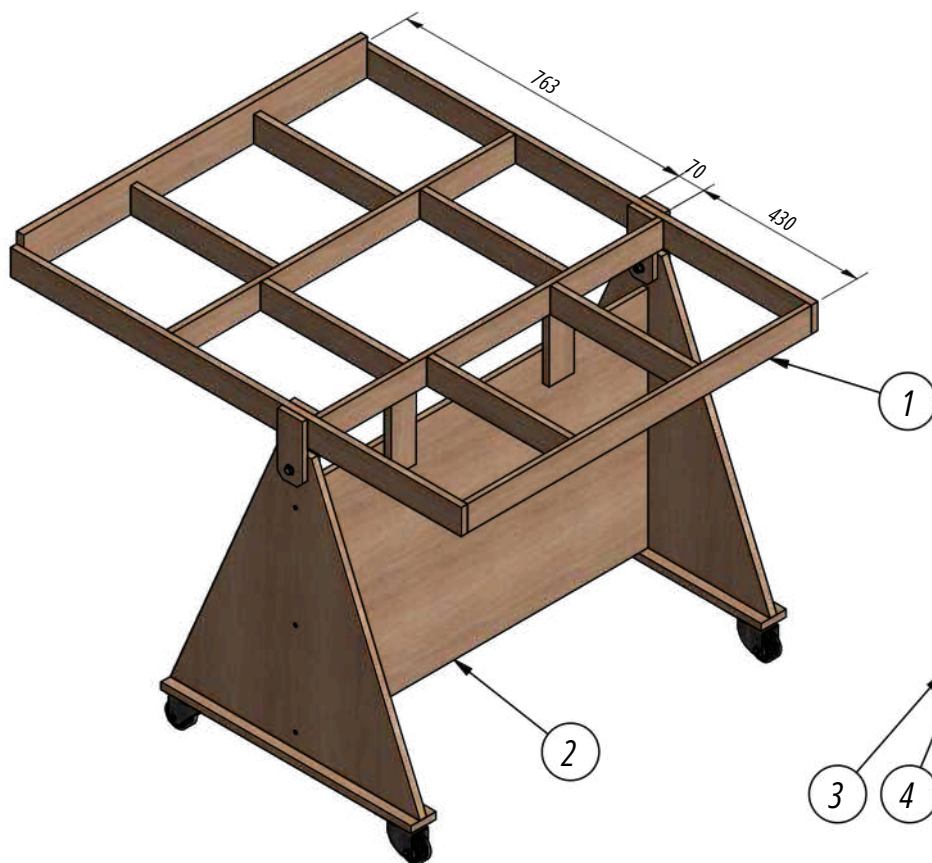
VISTA ISOMÉTRICA
