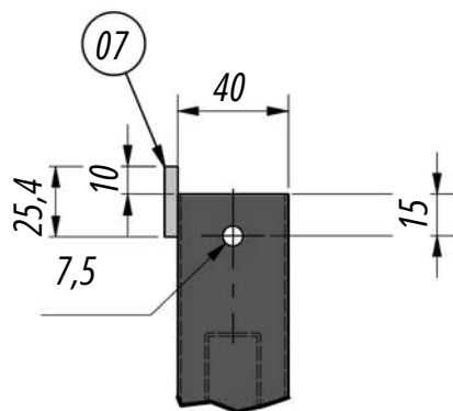
DET. FURAÇÃO
