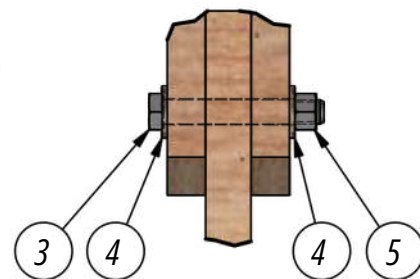
DET. FIXAÇÃO
