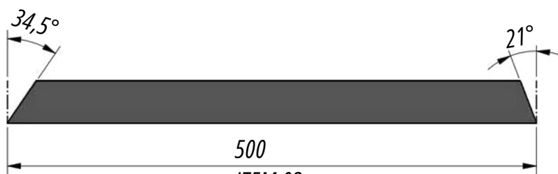
ITEM 03
