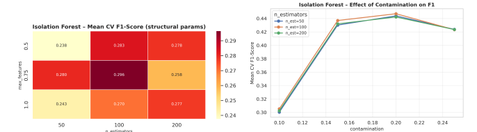
Fig. 4. Left: IF structural tuning mean CV F1 heatmap. Right: Validation F1 threshold sweep across candidate contamination values.
