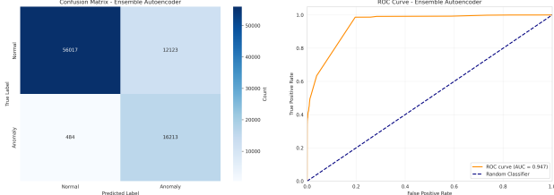
Fig. 9. Left: Ensemble Autoencoder Confusion Matrix. Right: Ensemble Autoencoder ROC Curve (AUC = 0.947).
