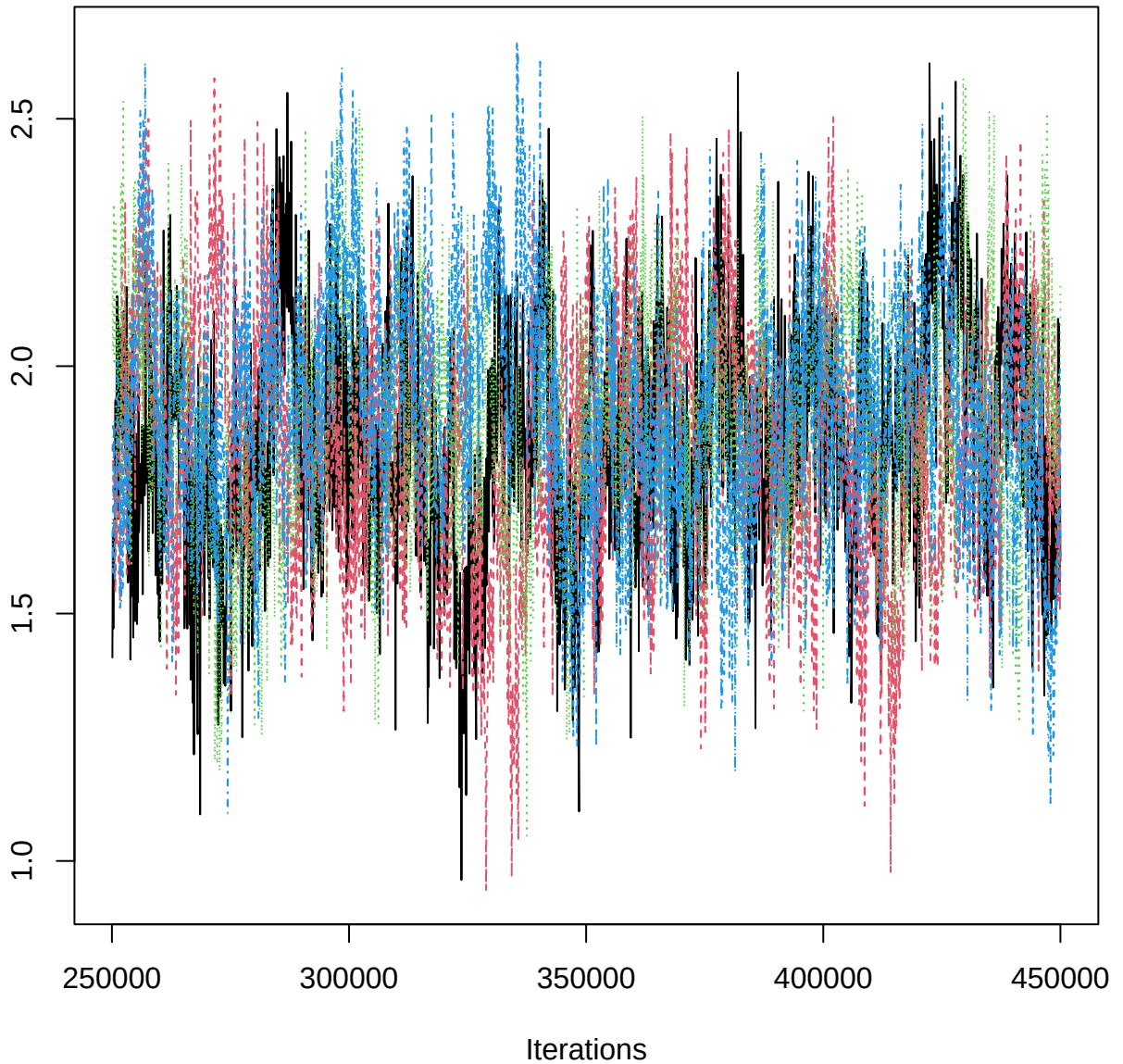
Traceplot – B[rtp (C7), ERS_n (S2)]
