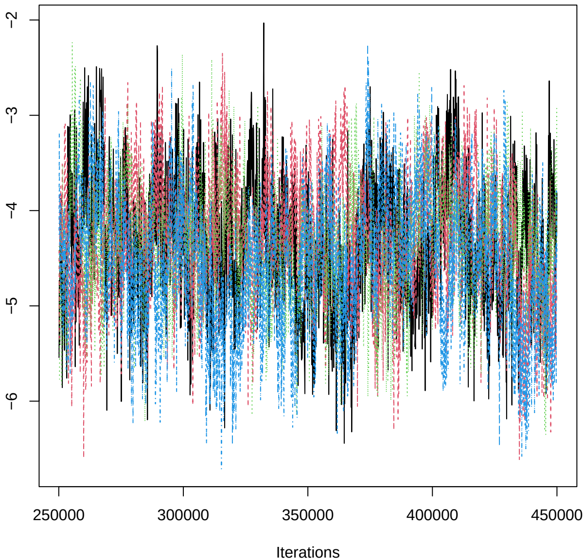
Traceplot – B[pH (C4), ERS_n (S2)]
