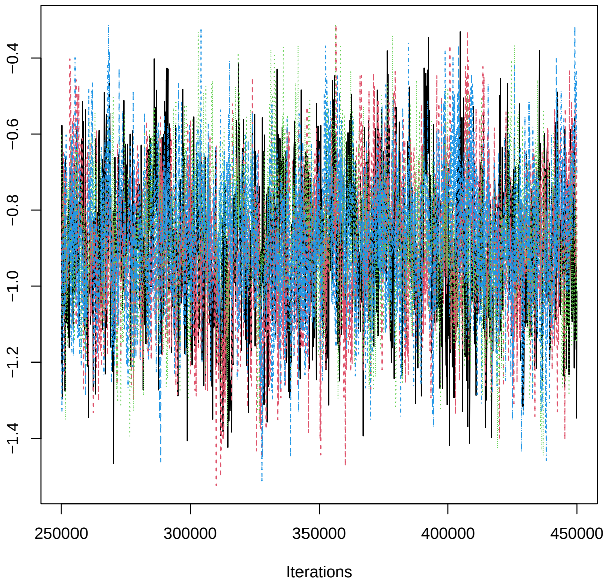
Traceplot – B[rtp (C7), EPB_n (S6)]
