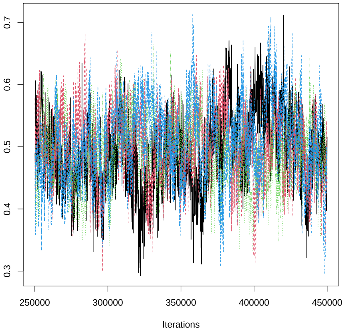
Traceplot – B[OM (C6), ERS_n (S2)]
