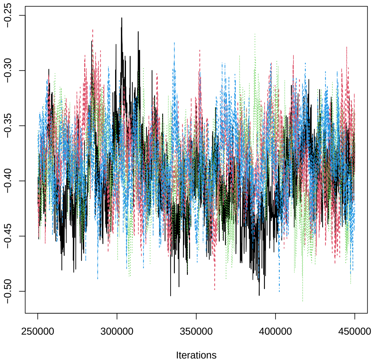
Traceplot – B[twi (C8), ERS_n (S2)]
