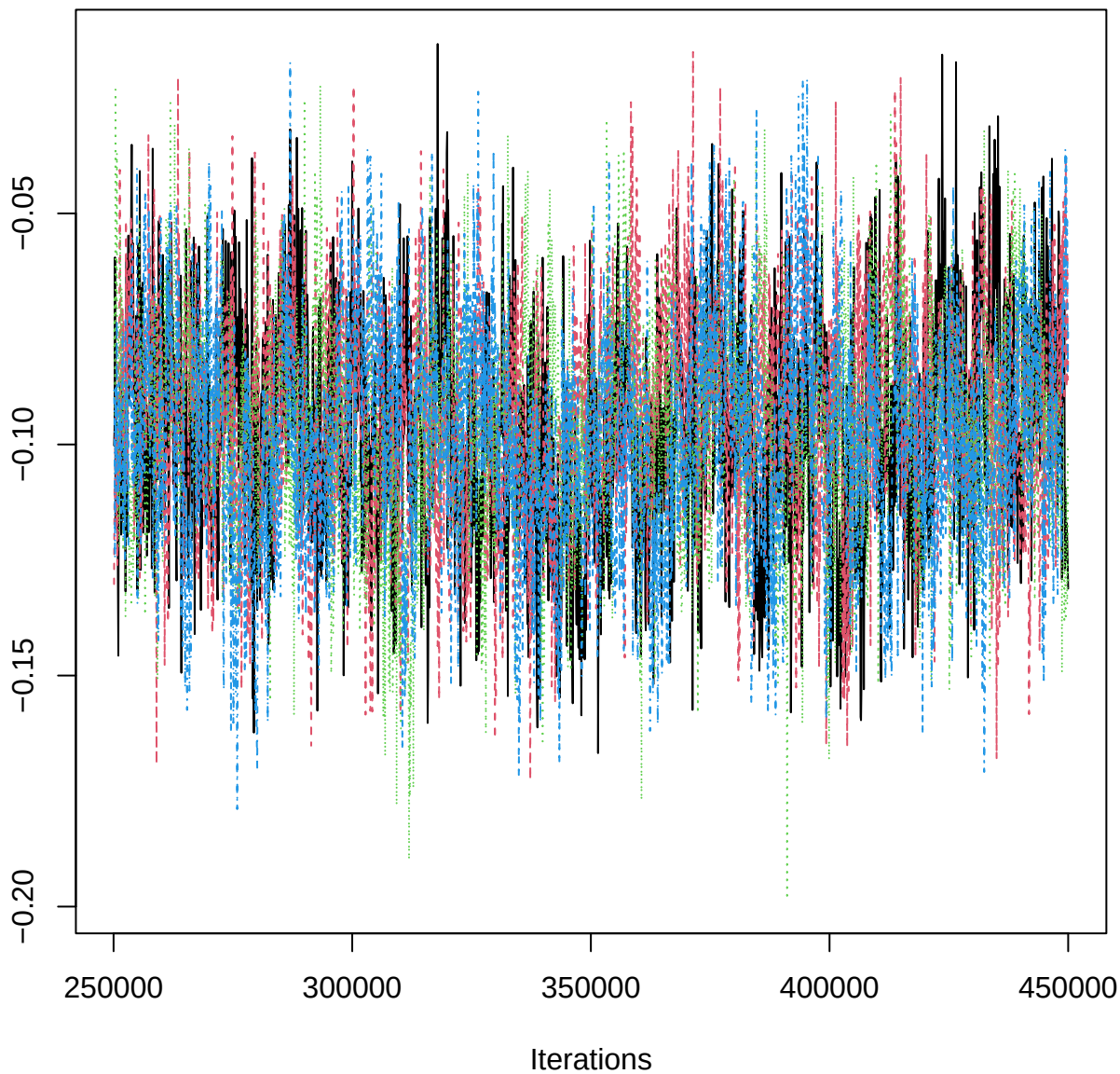
Traceplot – B[twi (C8), EPB_n (S6)]
