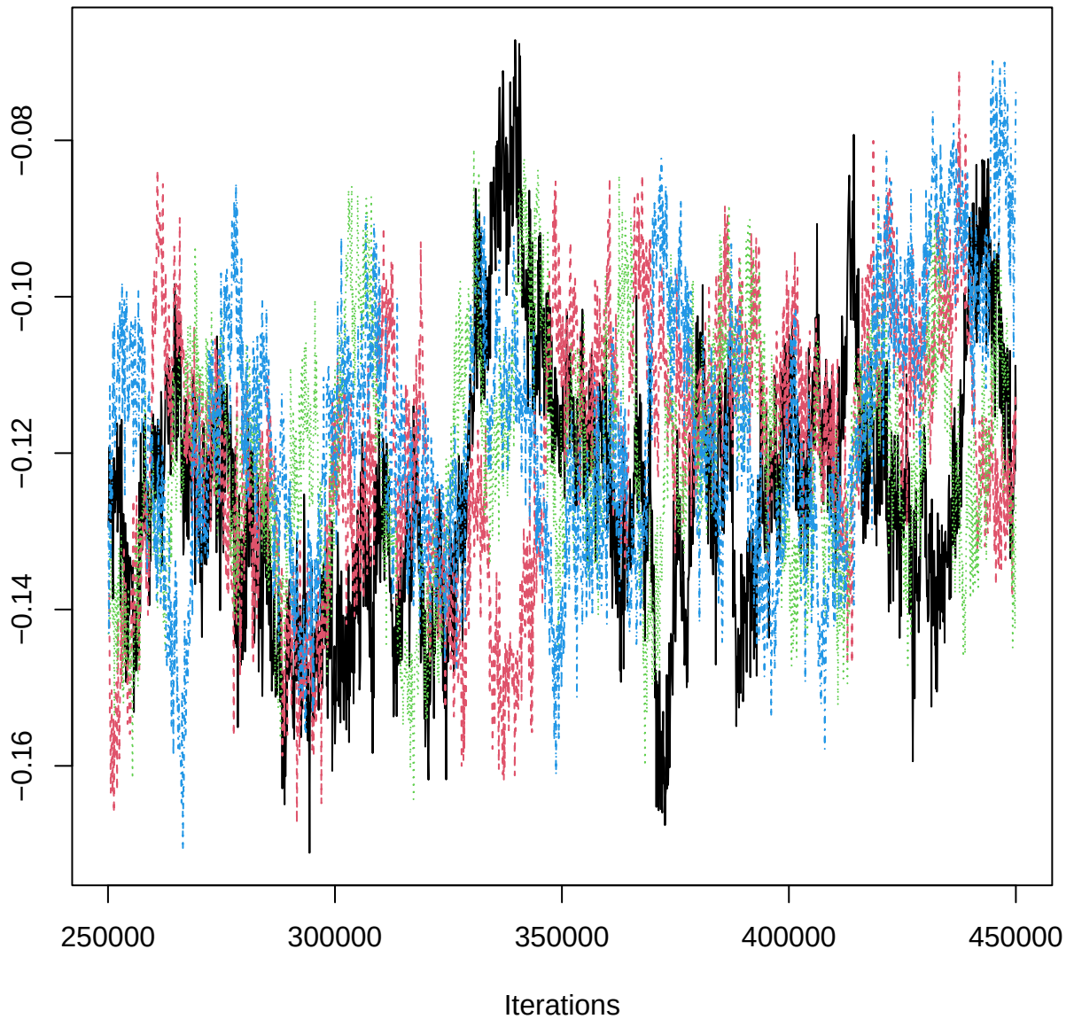
Traceplot – B[Clay (C5), ERS_n (S2)]
