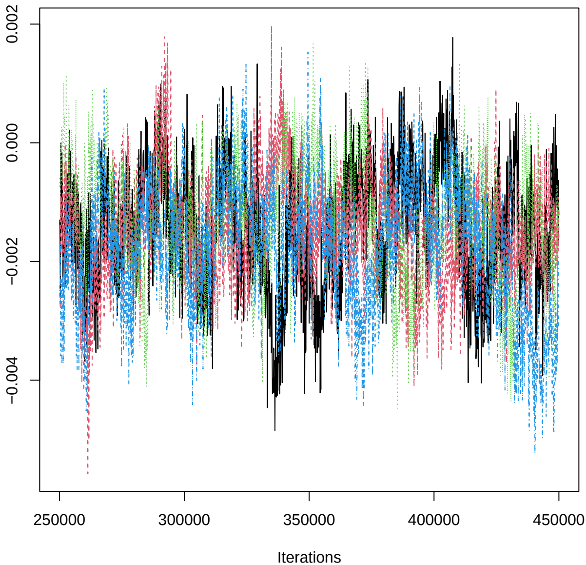
Traceplot – B[MAP (C2), ERS_n (S2)]
