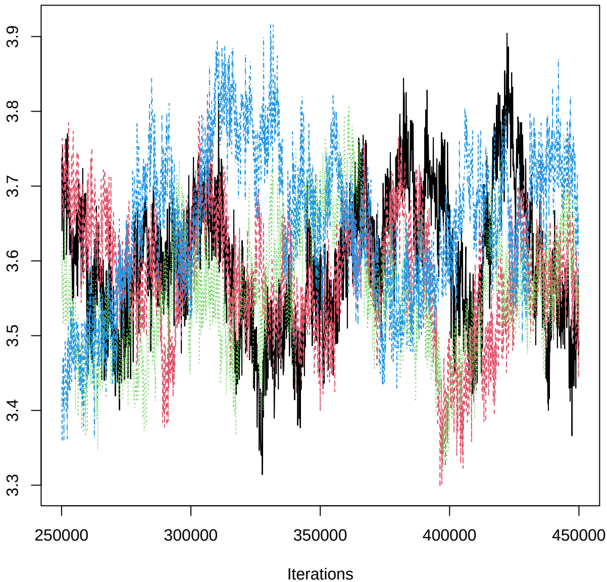
Traceplot – B[MAT (C3), ERS_n (S2)]
