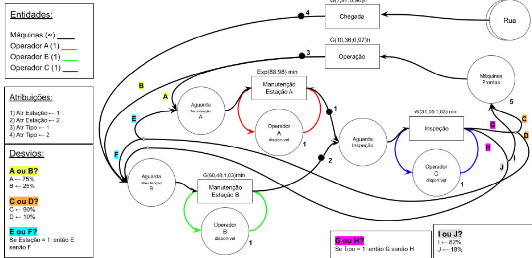
Figura 2: DCA do fluxo de manutenção de máquinas internas e externas
