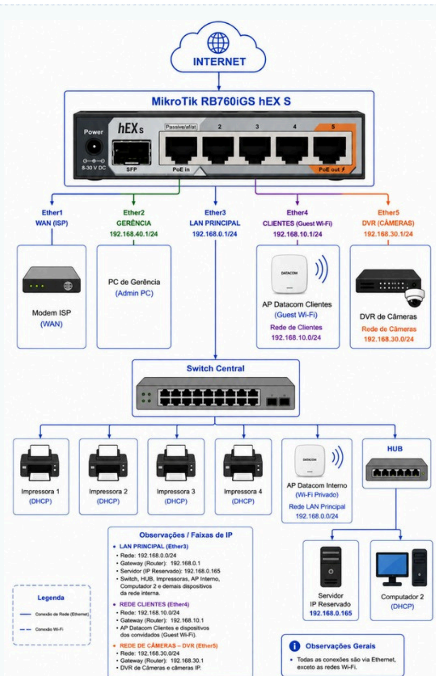
Figura 1: Diagrama de Fluxo Lógico e Segmentação de Sub-redes (MikroTik RB760iGS hEX S).
