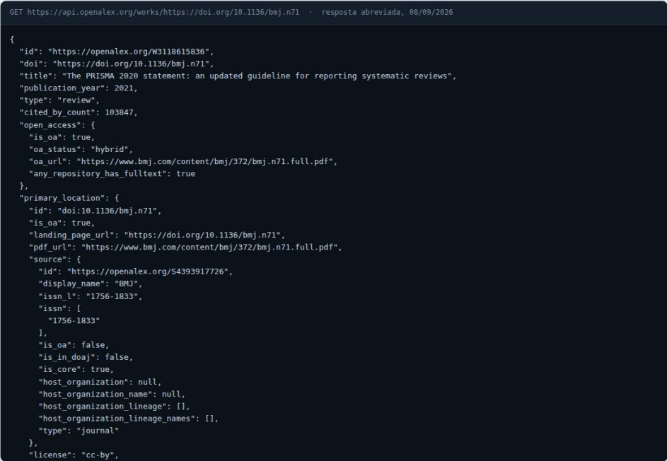
FIGURA 5 Captura real, 08/09/2026: a resposta da API aberta da OpenAlex para um DOI (o artigo do PRISMA 2020), com título, ano, contagem de citações, status de acesso aberto e URL do PDF — tudo que uma triagem precisa para enriquecer um registro, sem custo e por script.
