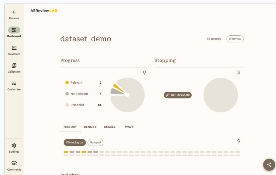
FIGURA 11 Dashboard após seis rótulos: 2 relevantes, 4 não relevantes, 54 por rotular; curvas de história, densidade e recall; e o bloco Stopping → Set Threshold.
