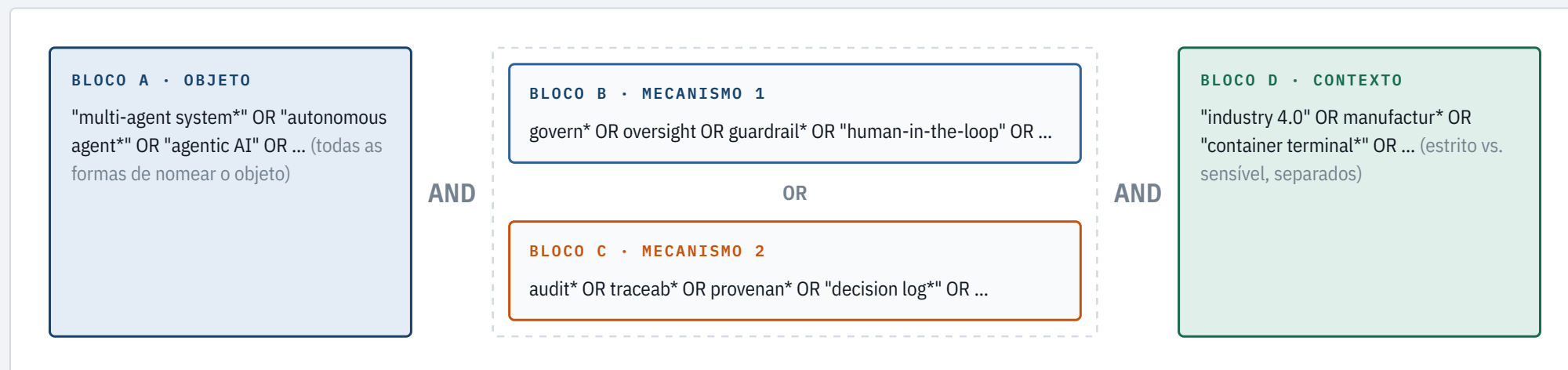
FIGURA 3 Estrutura A AND (B OR C) AND D. Dois detalhes de projeto: B e C se combinam por OR quando as perguntas não exigem coocorrência; e o bloco de contexto se divide em «estrito» e «sensível» — o segundo aumenta recall, mas não responde sozinho à pergunta do domínio.
