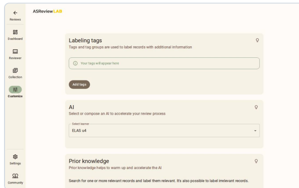
FIGURA 13 Customize: escolha do learner (aqui o padrão ELAS u4) e o conhecimento prévio — ao menos um registro relevante e um irrelevante, que o conjunto-semente fornece.
