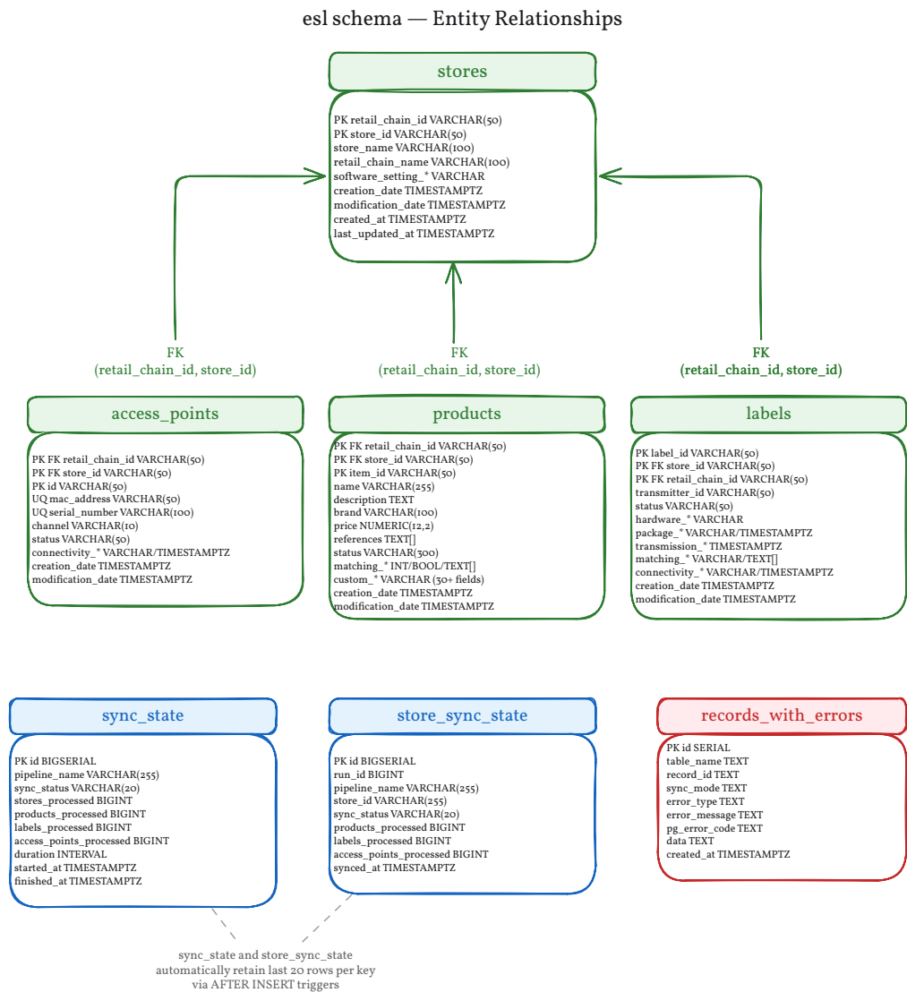
Figure 3: ER Diagram
