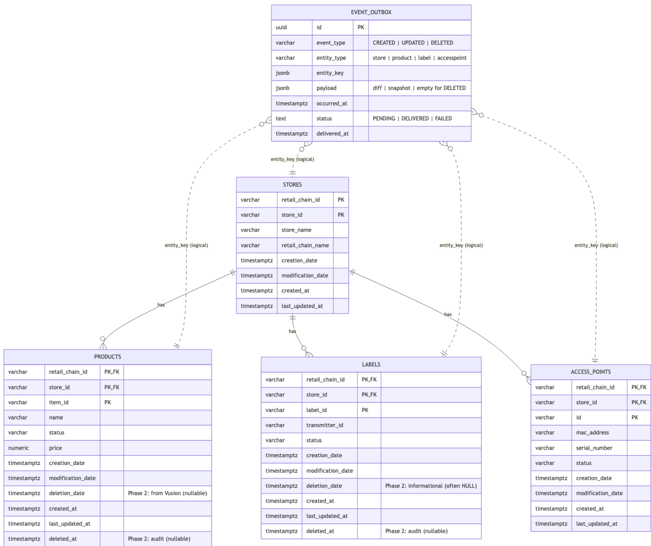
Figure 2: ER Diagram
