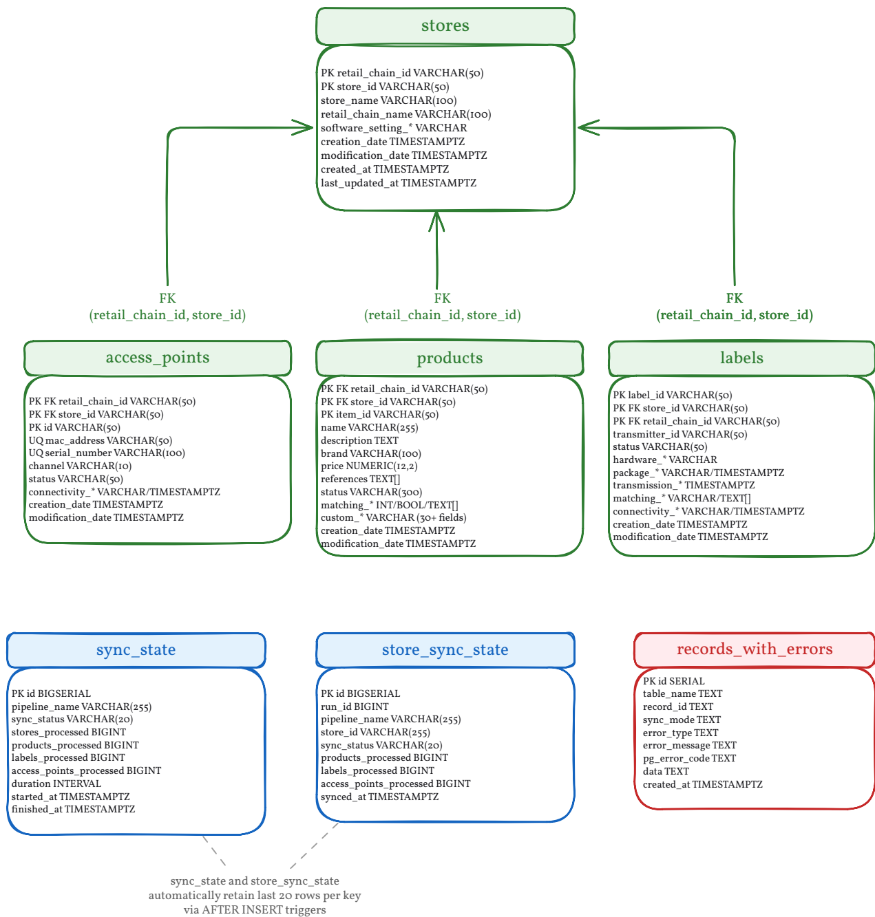
Figure 3: ER Diagram
