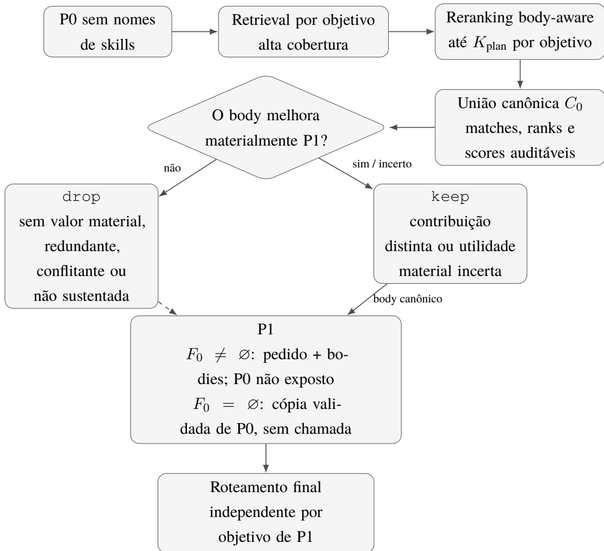
Figura 4 - Feedback pré-execução da MOSAIC 0.3
