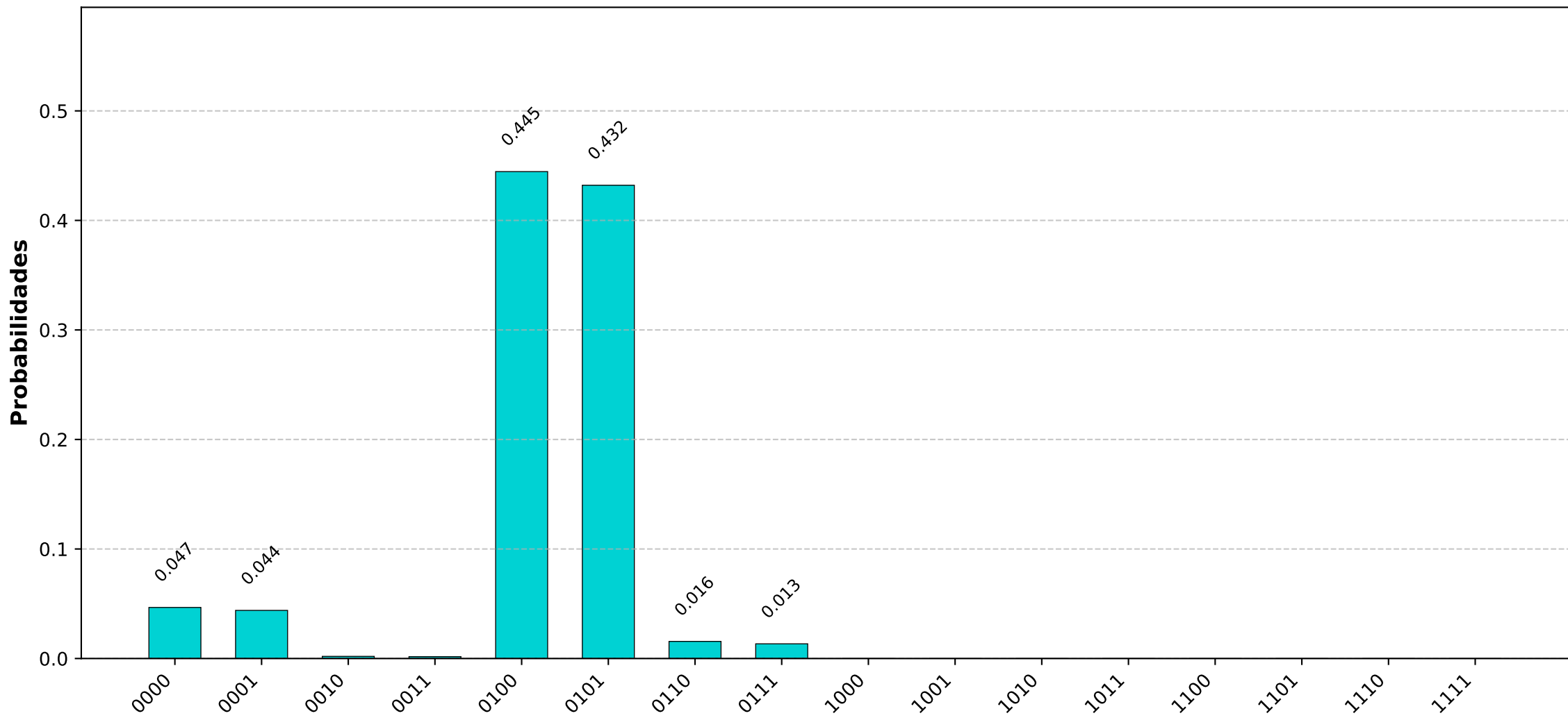
Cenário 5: Google Cirq
