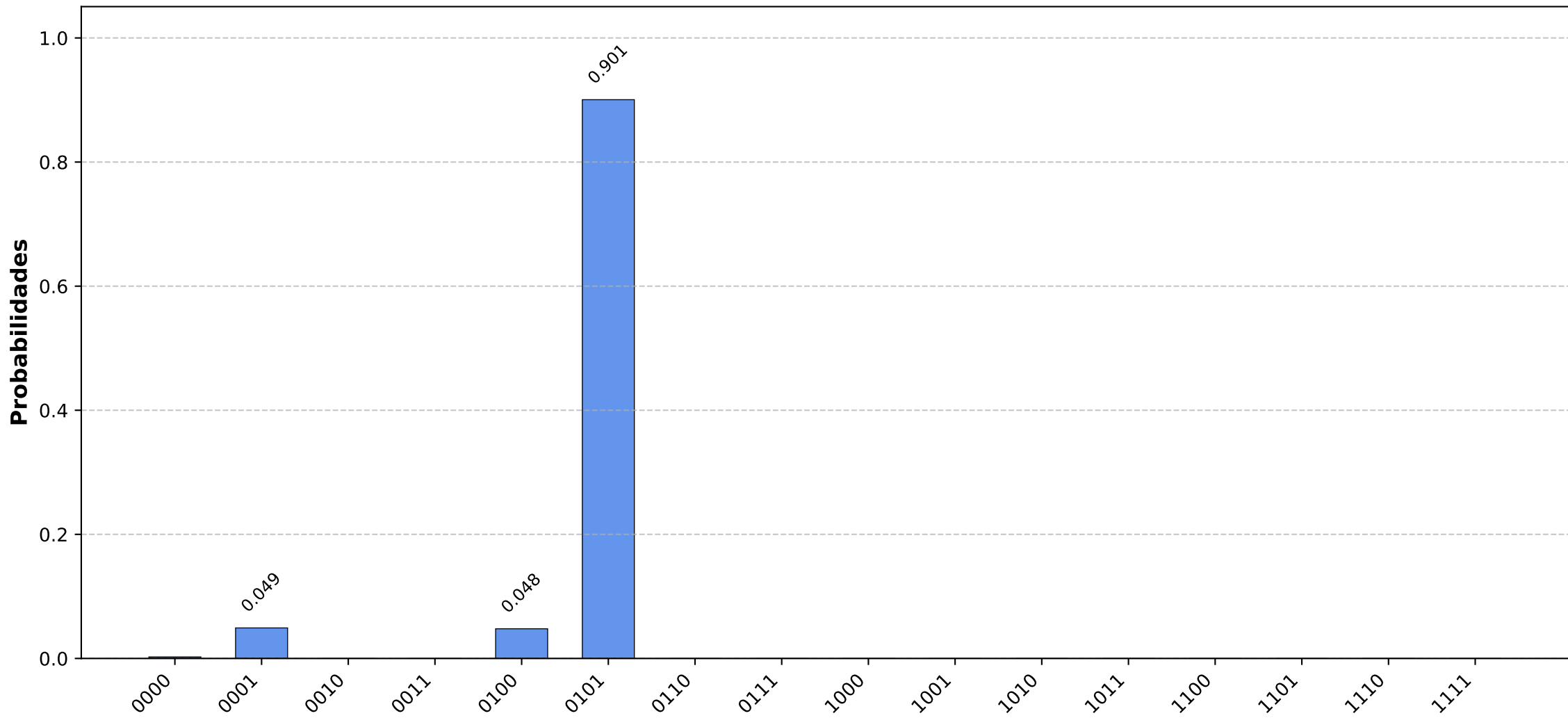
Cenário 3: Hardware Quântico Real NISQ (Sem Espião)
