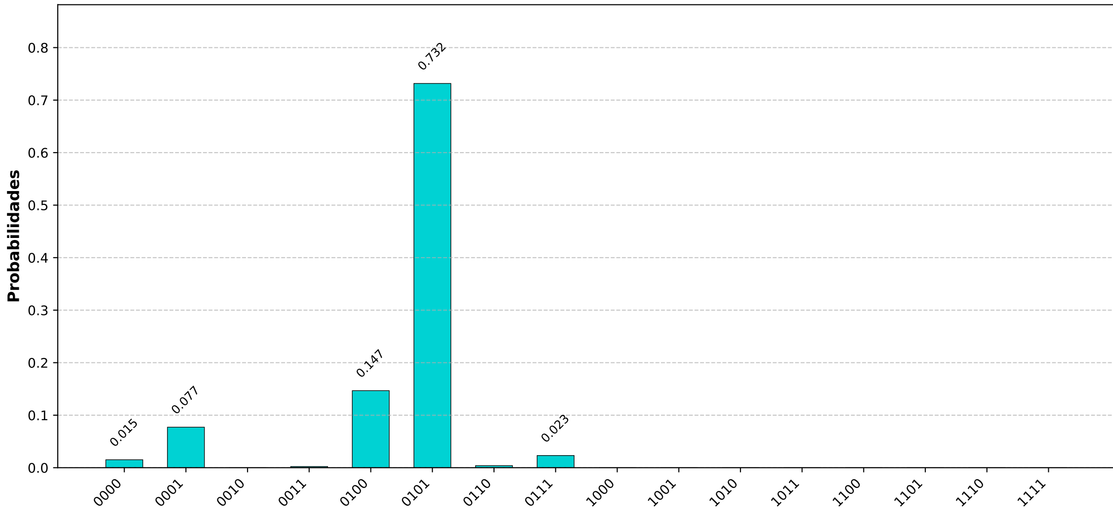
Cenário 5: Nossa Proposta Validada na Google (Cirq)
