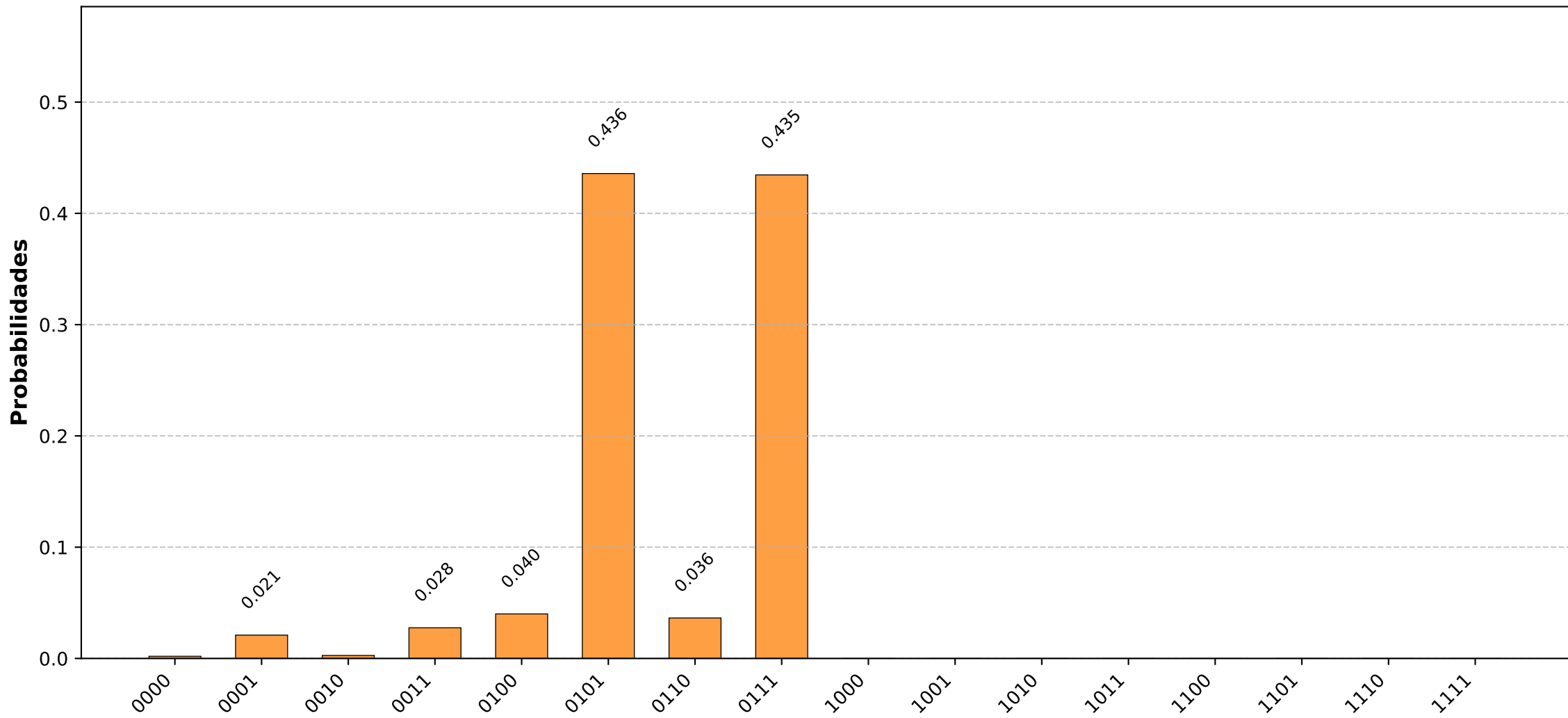
Cenário 4: Nossa Proposta - Simulador Ruidoso (Qiskit)
