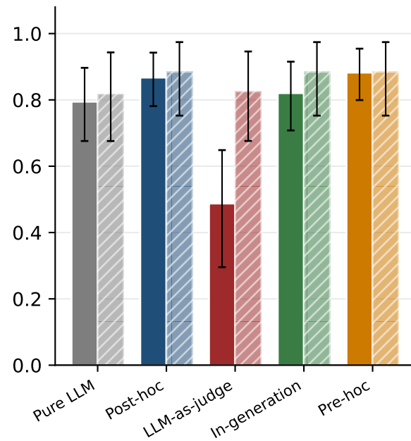
AC2 (linear)
