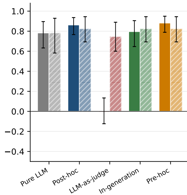
Kappa (quadratic)
