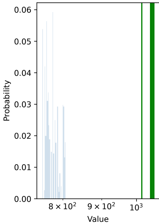
Posterior
