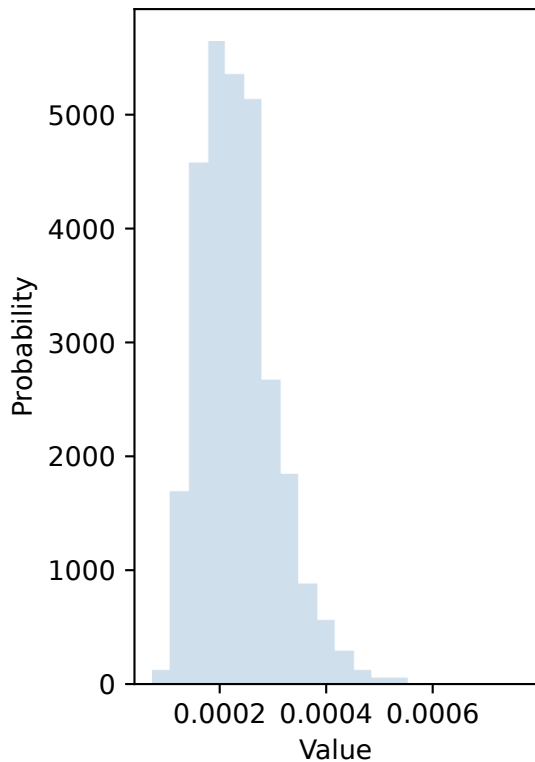
Posterior
