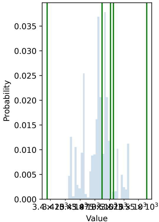
Posterior
