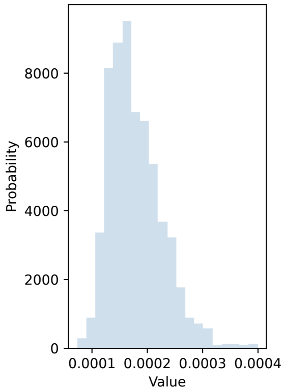
Posterior
