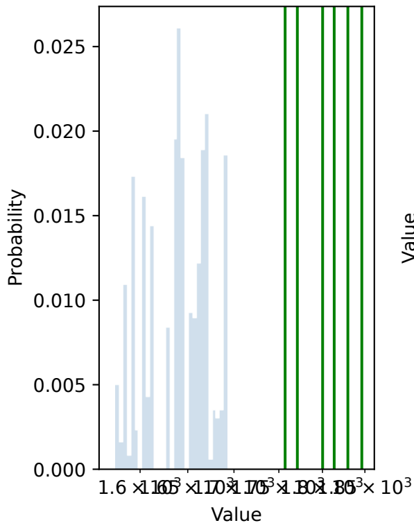
Posterior
