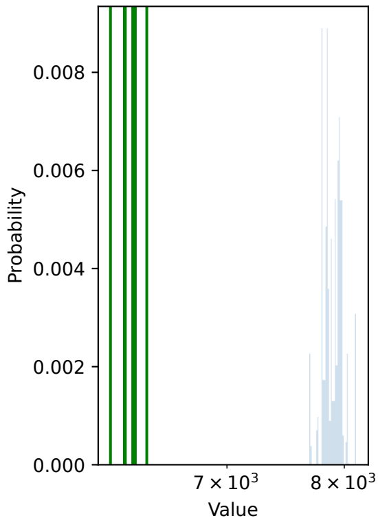
Posterior
