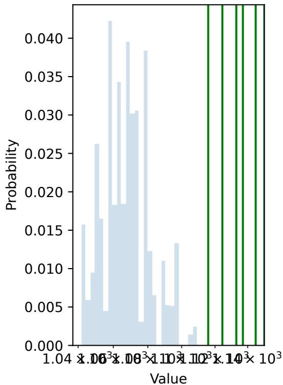
Posterior
